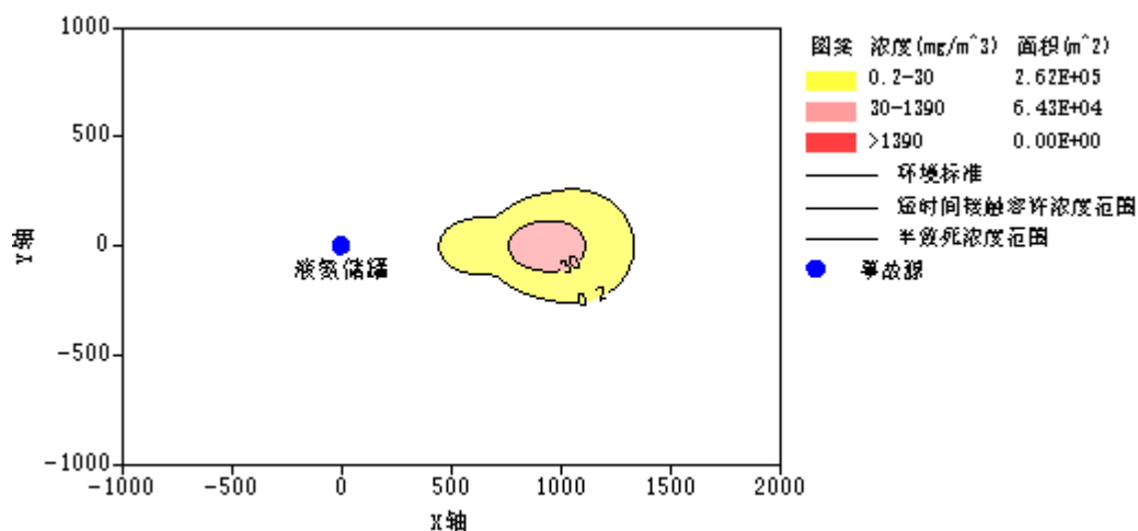
图表 0-4 公司液氨输送管泄漏 NH 3 浓度分布, 气象条件一, 5min
