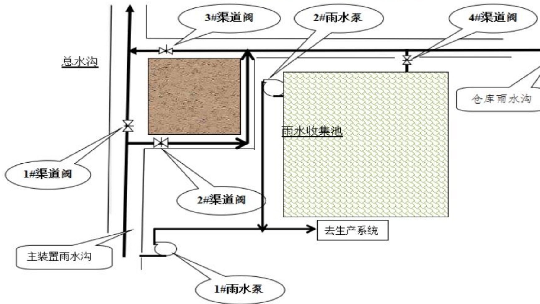
厂区雨水收集控制流程简图
