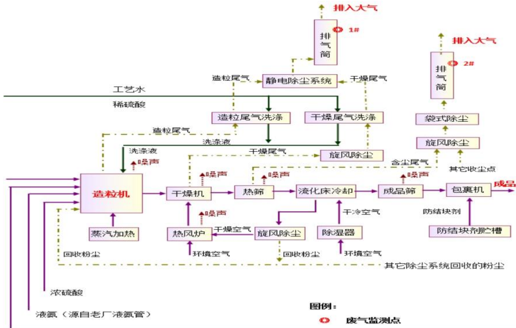
复合肥产污流程及废气监测点位图
