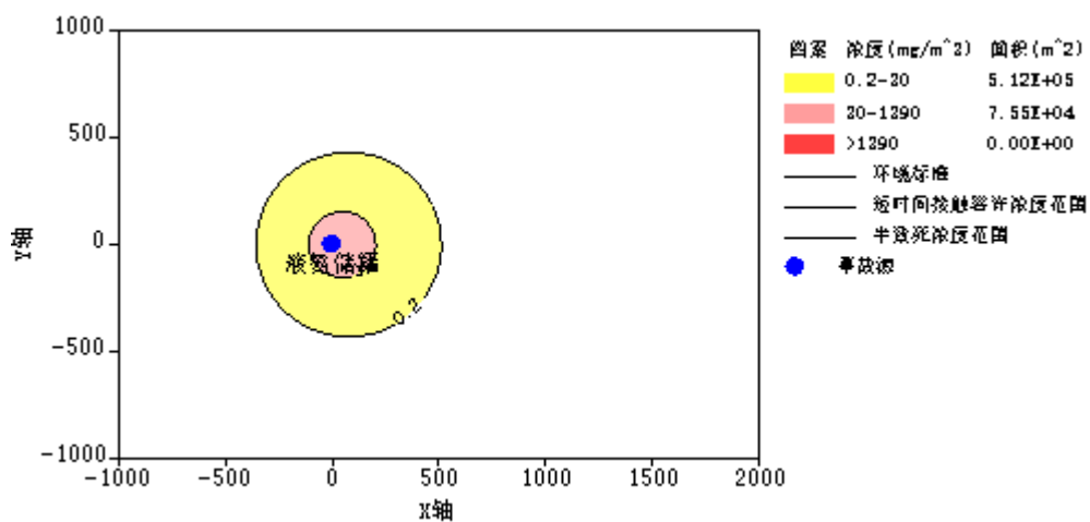
图表 0-5 公司液氨输送管泄漏 NH 3 浓度分布, 气象条件一, 15min
